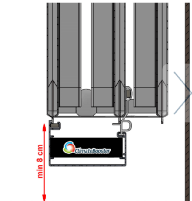
Bevestigingsprincipe 1 Type 33 - 2
