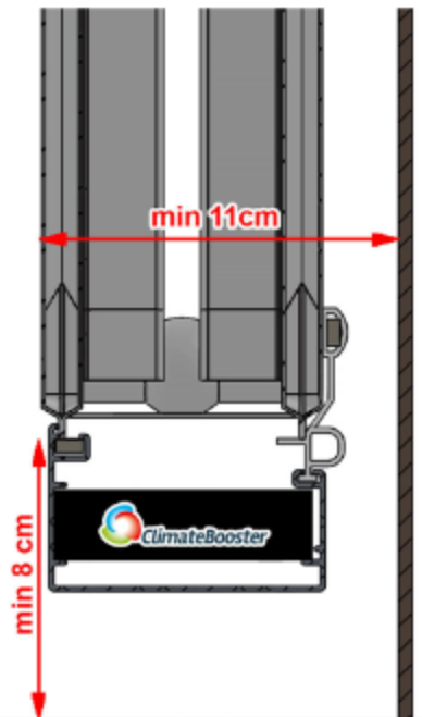
Bevestigingsprincipe type 20, 21 & 22
