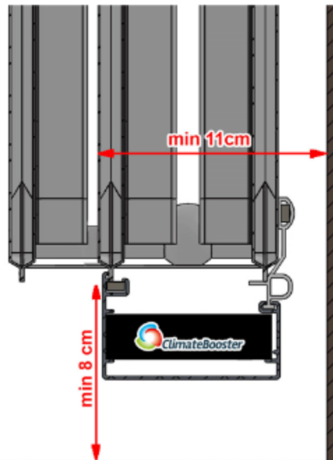
Bevestigingsprincipe Type 33 - 1
